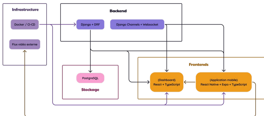
Schéma de la stack technique et architecture globale
